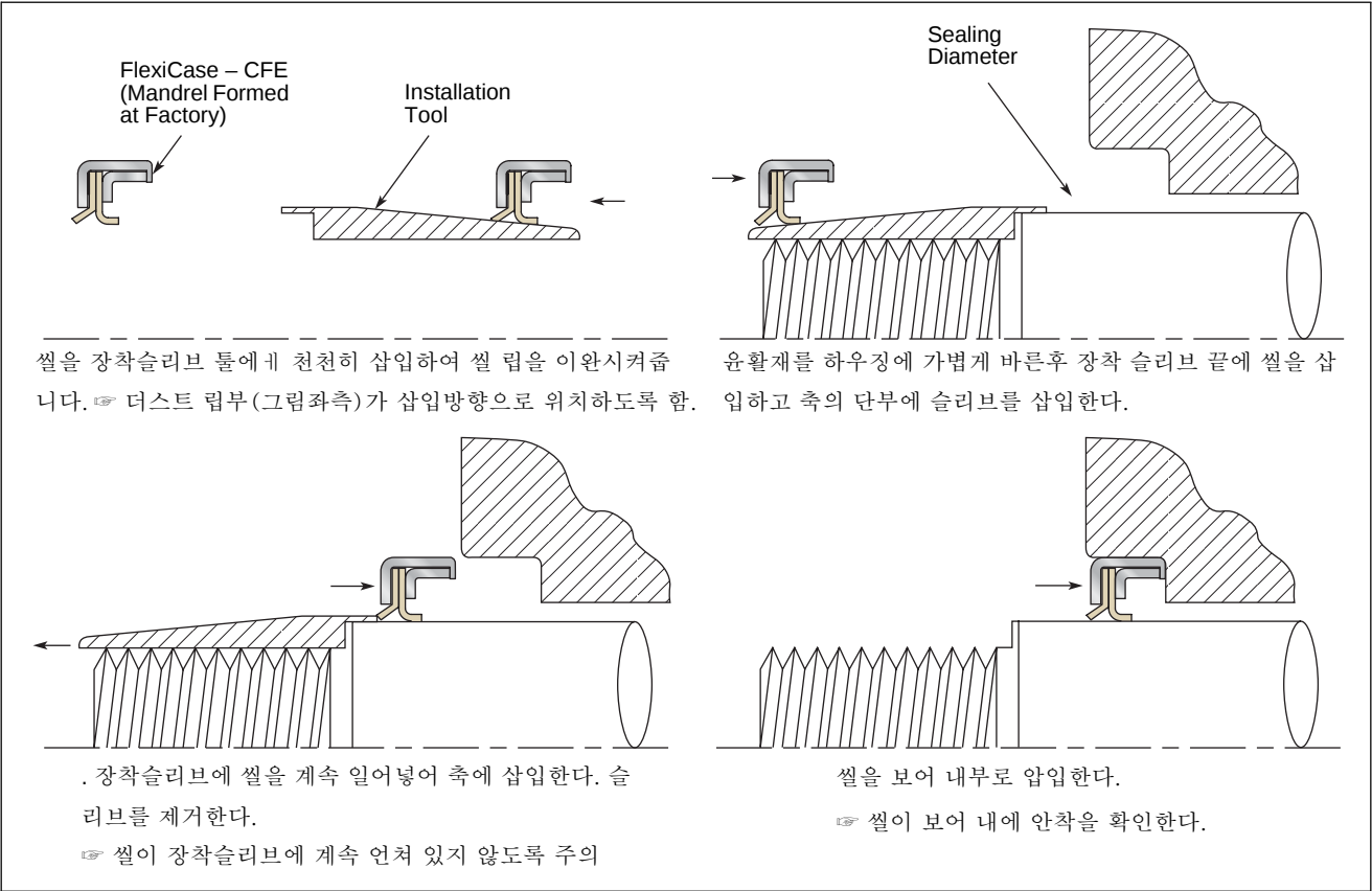
[메탈 케이스 테프론 립씰 장착 방법]
