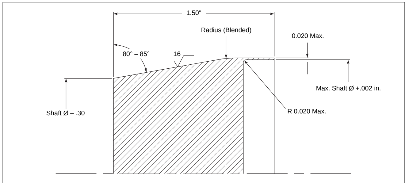
[ 일체형 테프론 립 셸 장착 슬리브 톨 형상및 치수 ]
